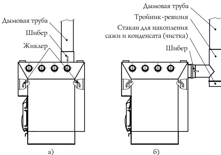
Рисунок 2. Схема присоединения котла к дымоходу.
