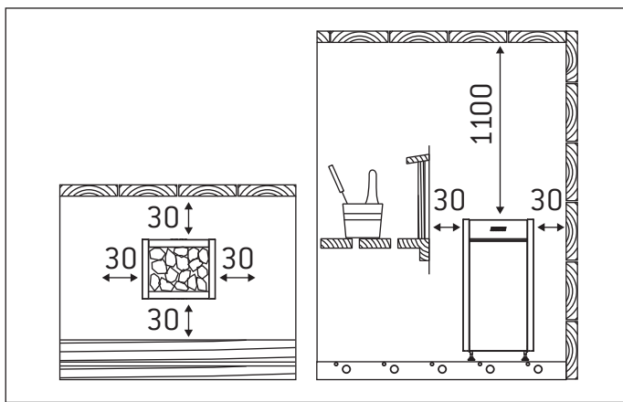
Kuva 4. Kiukaan suojaetäisyydet (mitat millimetreinä) Bild 4. Säkerhetsavstånd (måtten i millimeter)
